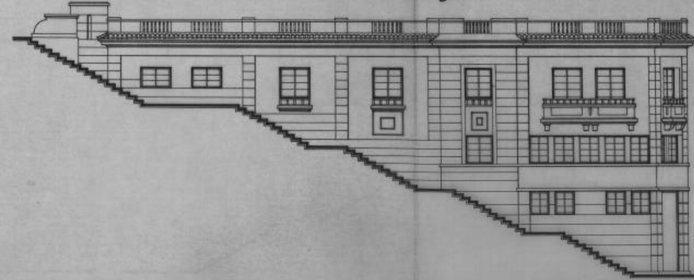
Fachada a escalinata en proyecto.
