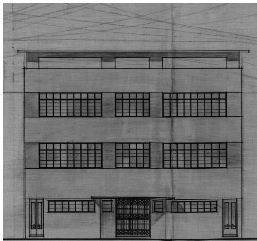
Reforma de fachada.
